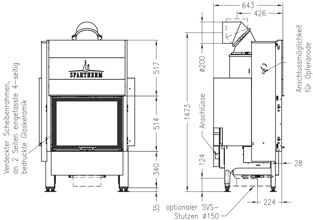
Vorderansicht front view M~1:20
